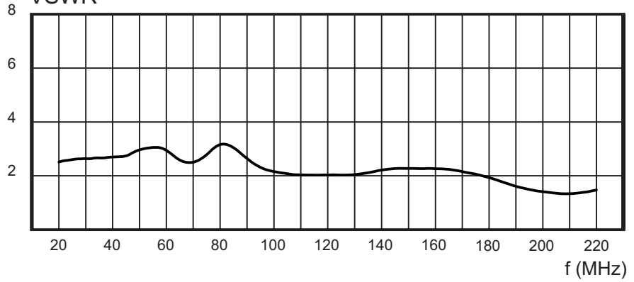
VSWR
