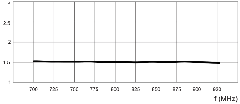
VSWR
